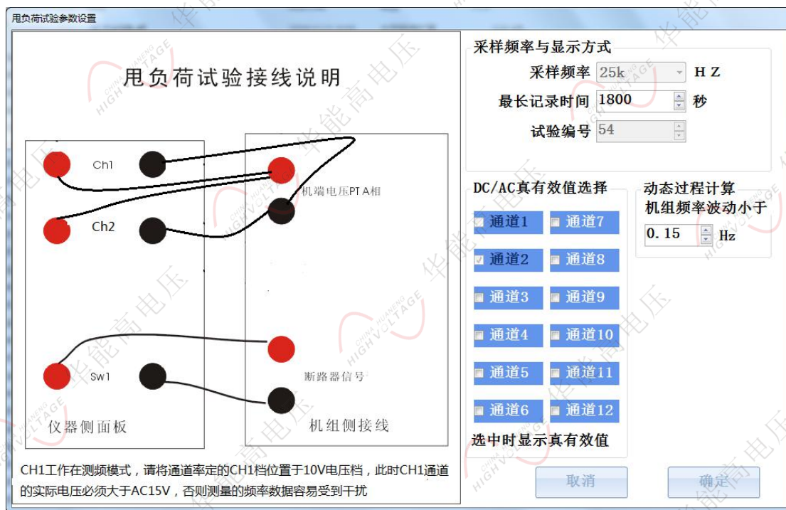
图 34 甩负荷试验参数设置
