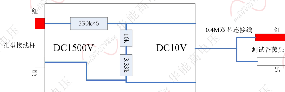
图 1 DC1500V/DC10V 变换器电气原理图
