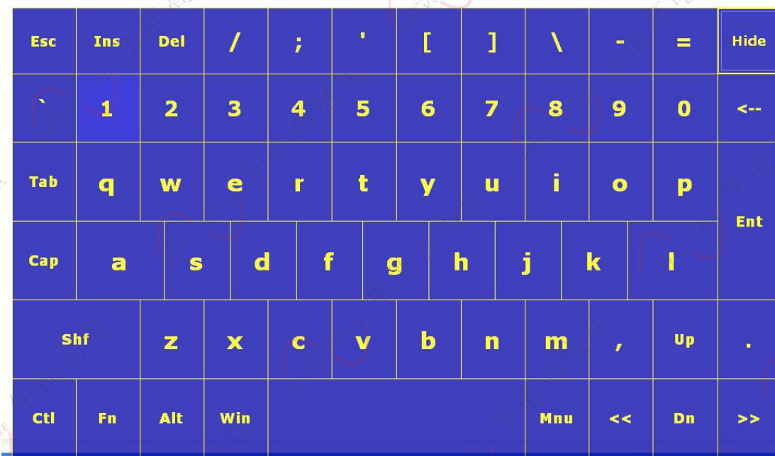
图 8 虚拟键盘
