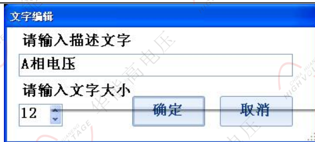
图 25 标识设置
