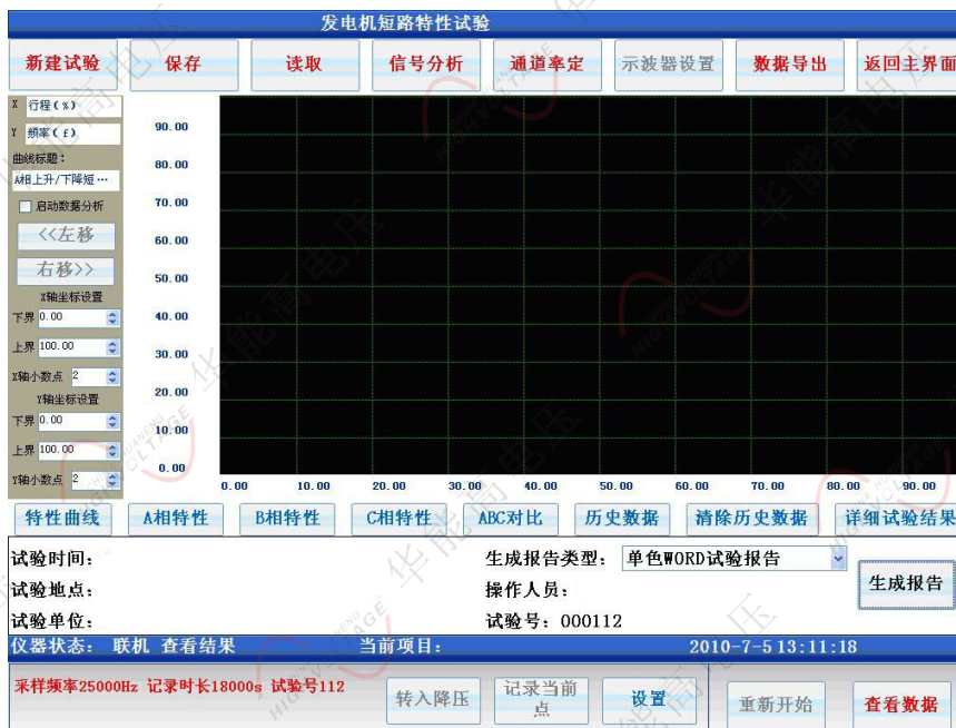
图 33 发电机三相短路特性曲线试验结果展示
