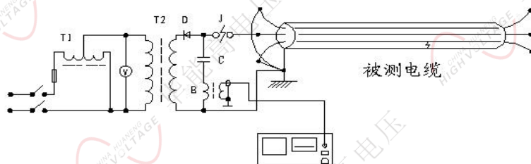
冲闪法电流取样接线图
