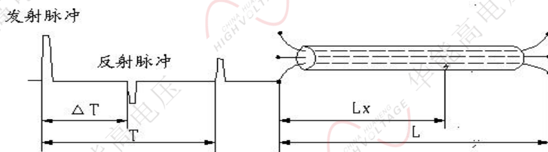
低压脉冲测试原理图
