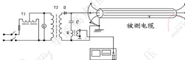
直闪法电流取样接线图
