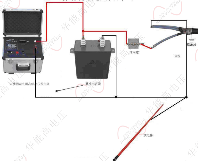
精确定点接线图(二)
