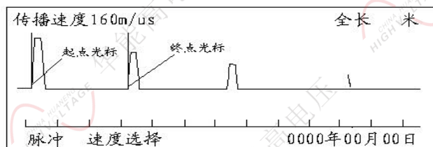
低压脉冲测全长波形(终端开路)
