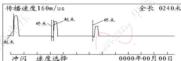
冲闪法电流取样测试波形
