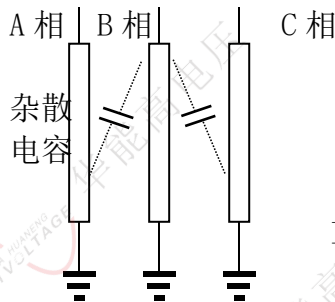
图十二、一字排列避雷器
