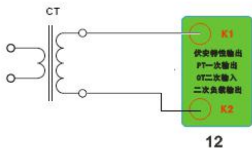
2. 接线图：图二 （CT 变比接线图）
