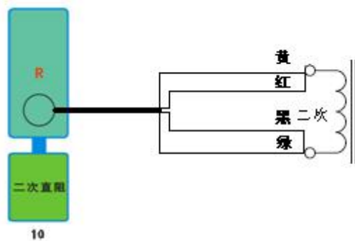
7. 接线图：图七 （二次直阻接线图）
