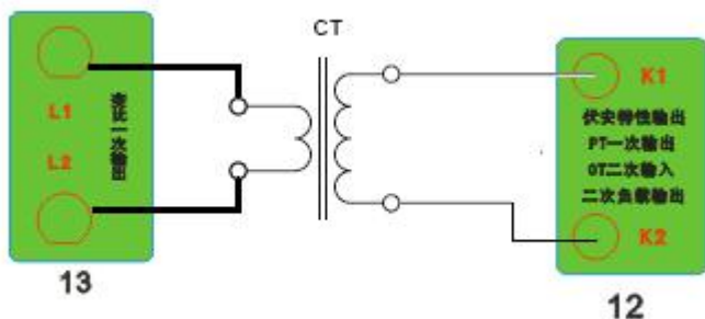
3. 接线图：图三 （二次回路接线图）
