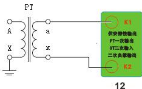
5. 接线图：图五 （PT 变比接线图）
