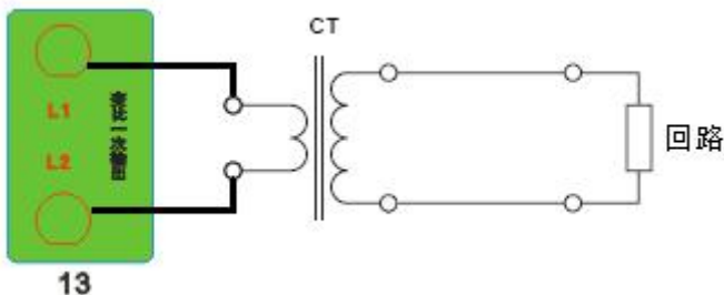
4. 接线图：图四 （PT 伏安接线图）
