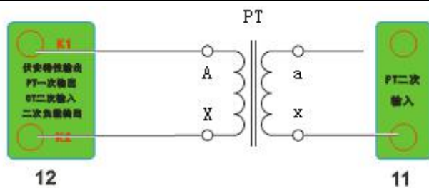
6. 接线图：图六 （二次耐压接线图）
