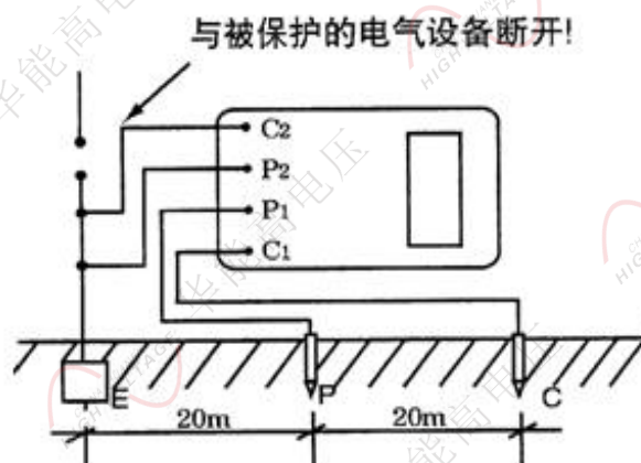
图 6 地桩法测量
