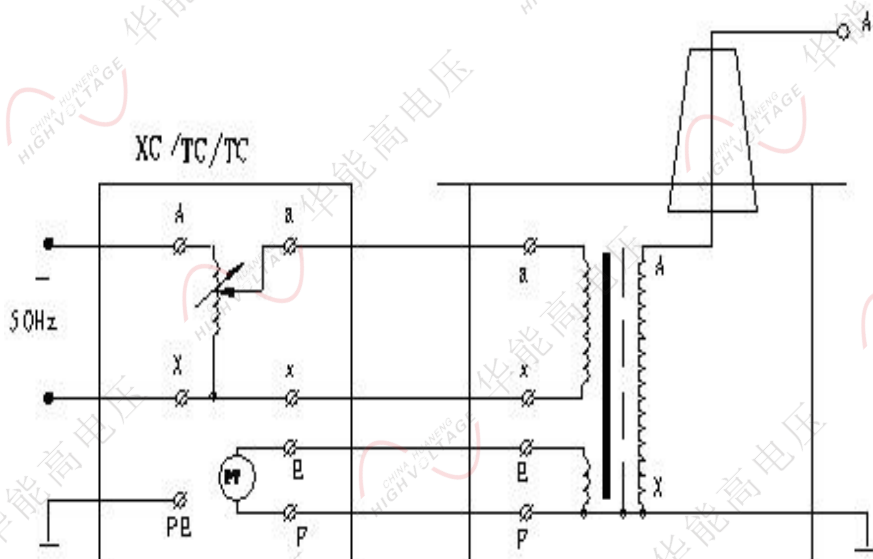
图 3：单台 HNYD 试验变压器原理图
