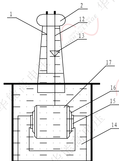
图 2：单台试验变压器内部结构图
