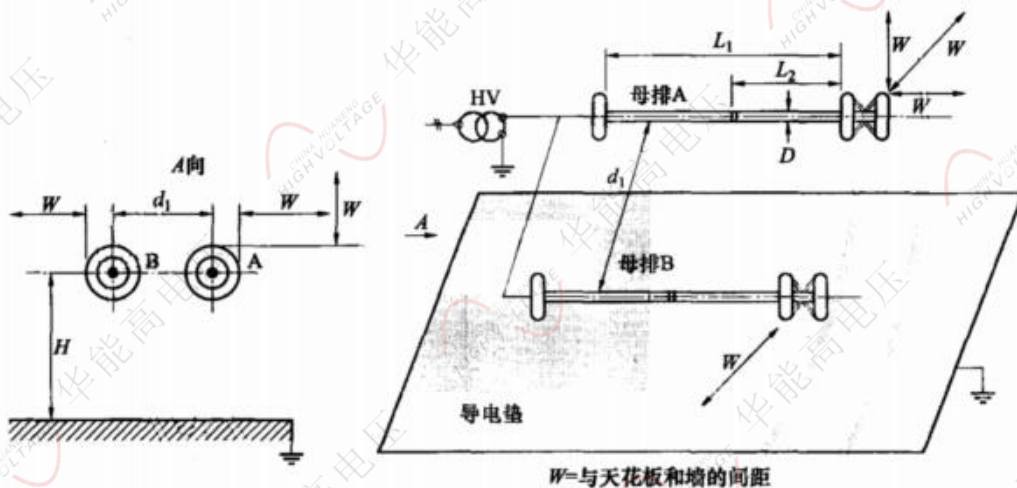
图5 试验布置图
