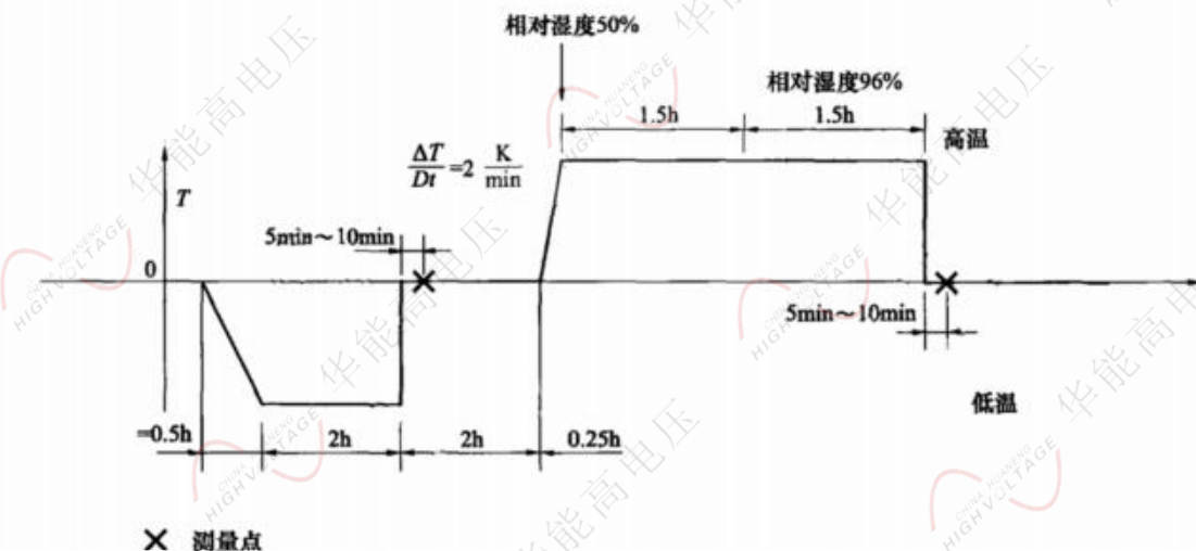
图 28 试验周期与气候的关系曲线
