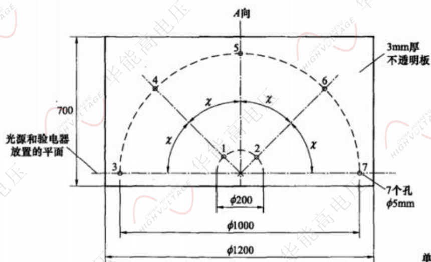
图 15 光指示信号的清晰可辨性试验布置
