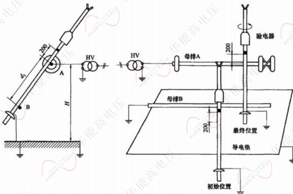
图 21 平行母线电极布置的沿面耐压试验
