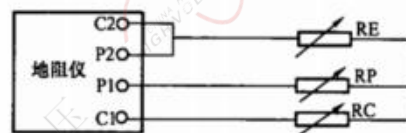
P1、P2—电压（电位）极端子；C1、C2—电流极端子； RE—标准器（等效接地电阻）；RP、RC—等效辅助接地电阻
