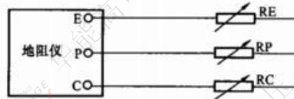
E—接地体端子；P—电压（电位）极端子；C—电流极端子； RE—标准器（等效接地电阻）；RC、RP—等效辅助接地电阻
