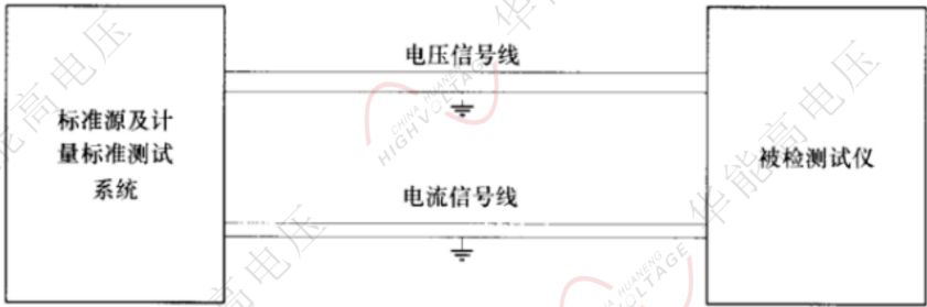
图 A.1 校验接线
