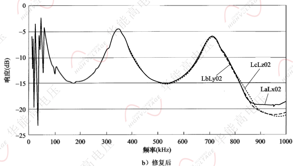
图 I.2 SFPSZ7-150000/220 变压器低压绕组变形时修复后的幅频响应曲线 (续)
