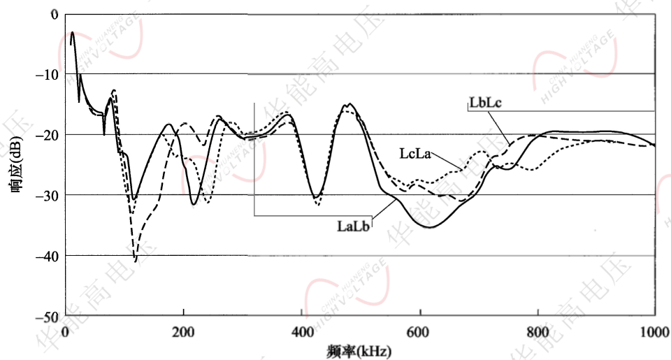
图 I.3 SFPS8-31500/110 变压器低压绕组变形时的幅频响应曲线
