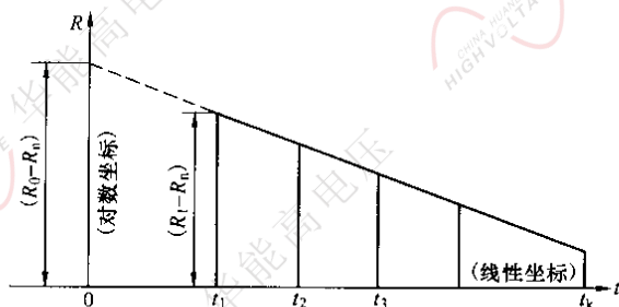
图 A.1 绕组温升测量计算 R_0 图
