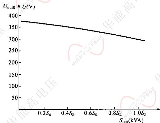
图 3 装置的输出电压特性曲线
