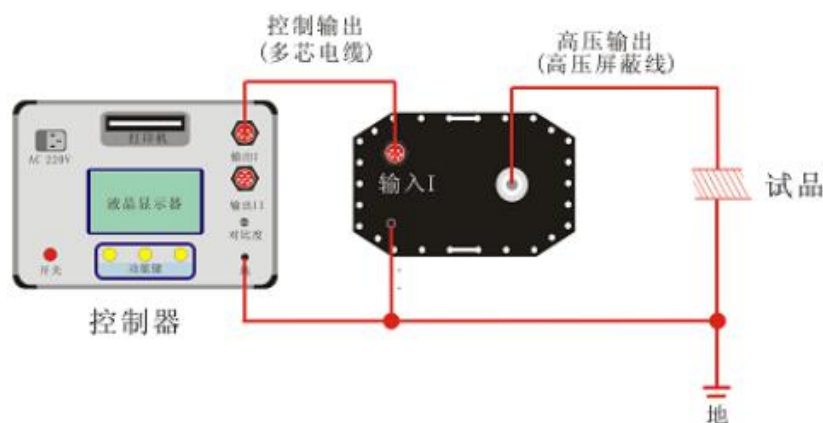
图 19 测量电容器的连线图
