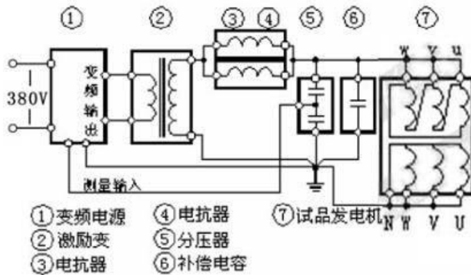
变压器耐压试验接线图
