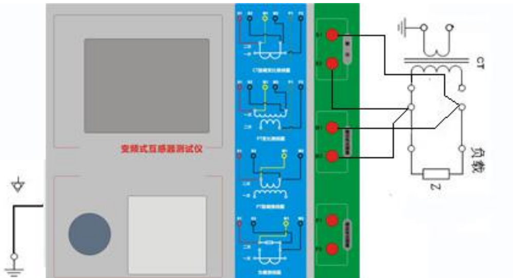
图 2.2 CT 二次负荷试验接线方式
