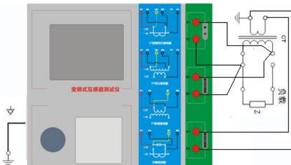
图 2.1 CT 直阻、励磁、变比试验接线方式
