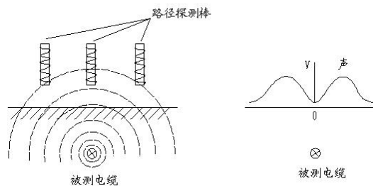
电缆路径探测原理图
