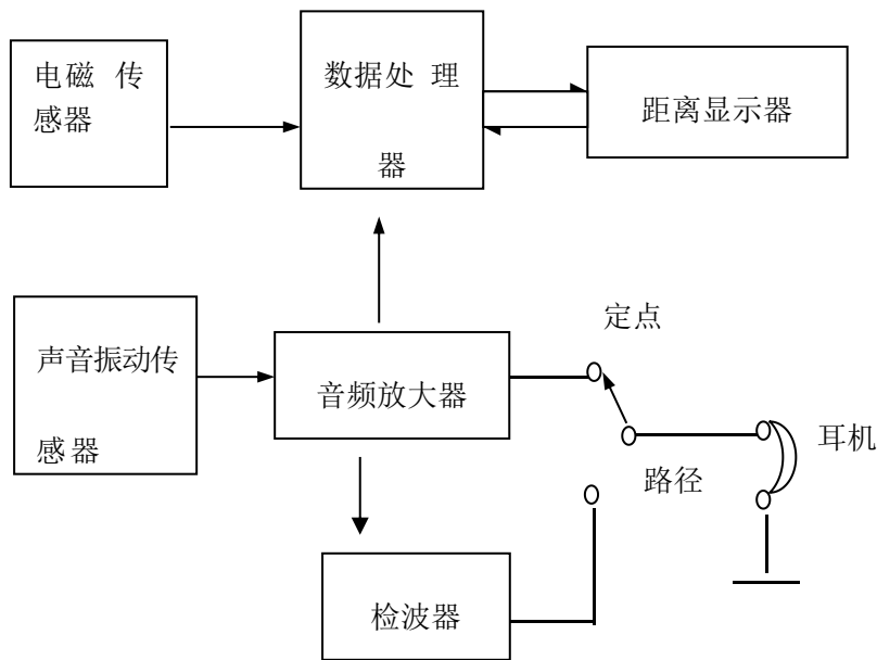
图 2 原理框图
