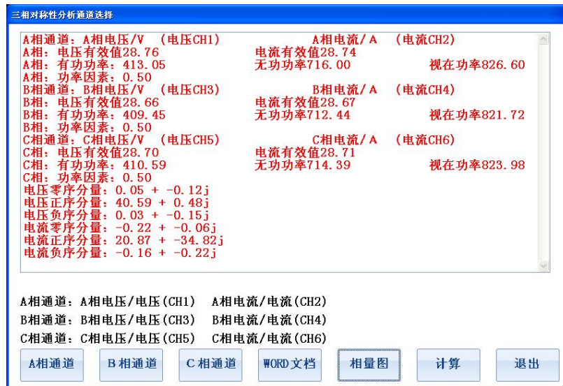
图 27 三相分析
