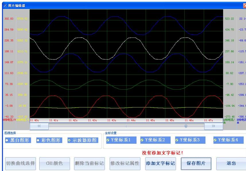
图 24 图形编辑
