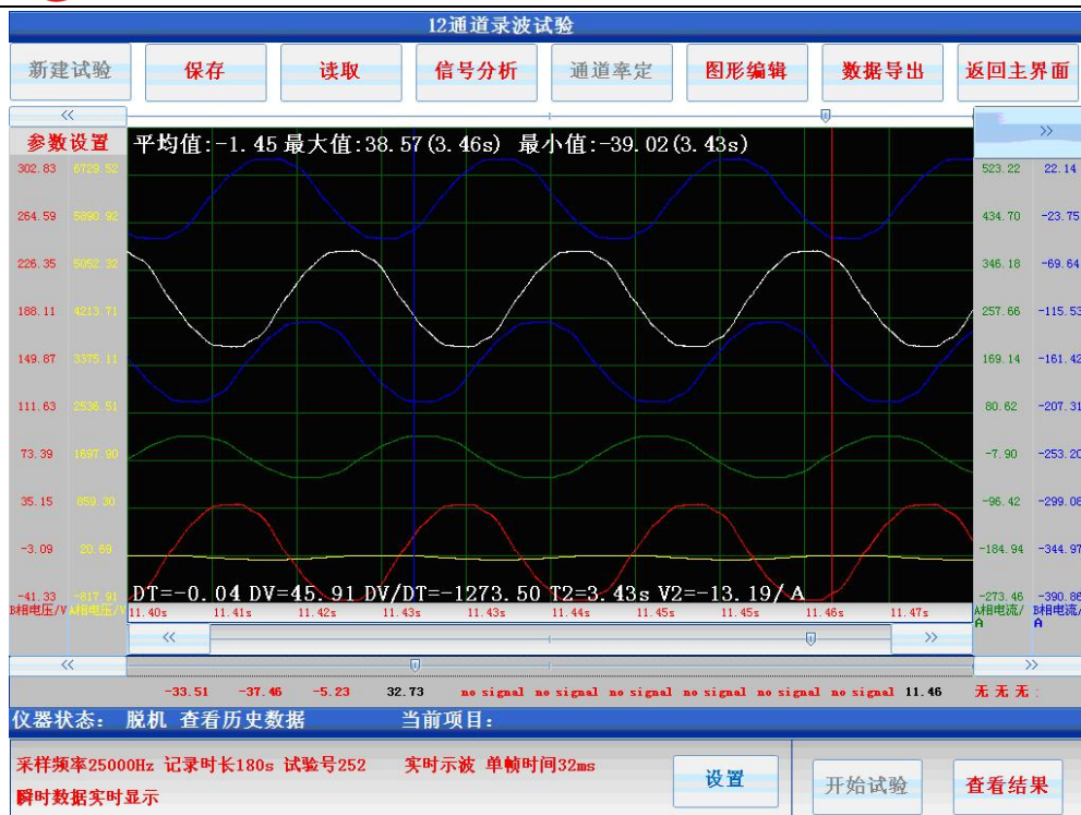
图 16 双线统计
